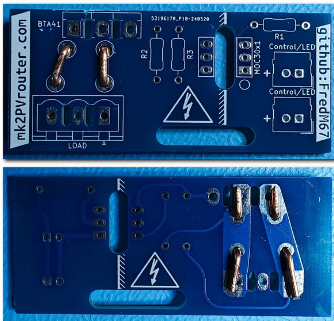
Vue dessus/dessous, agrafes posées
