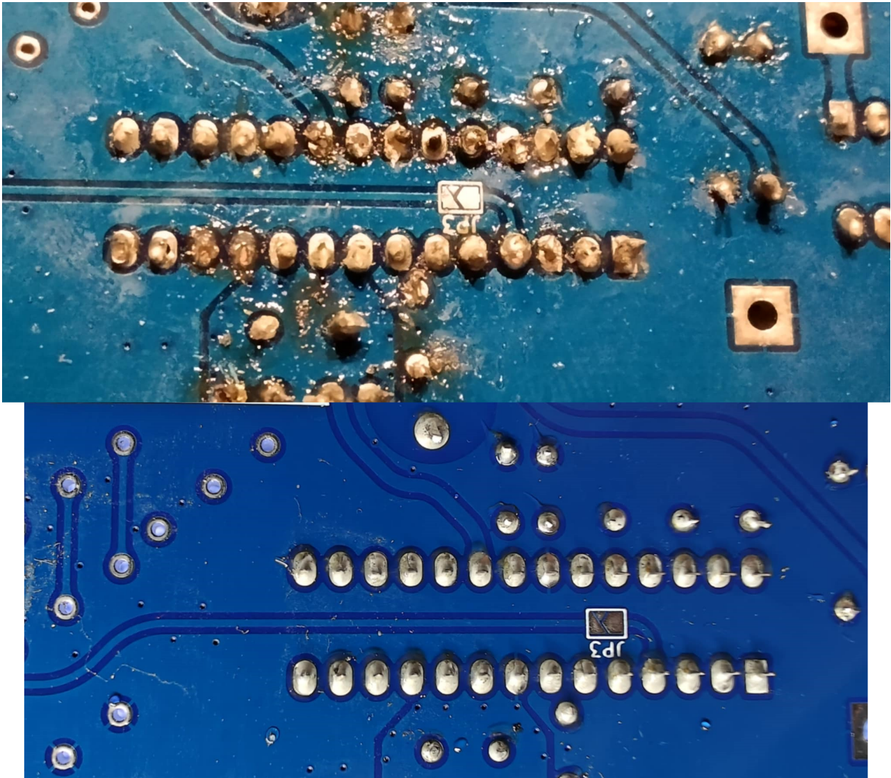
Exemples de bonnes et mauvaises soudures
