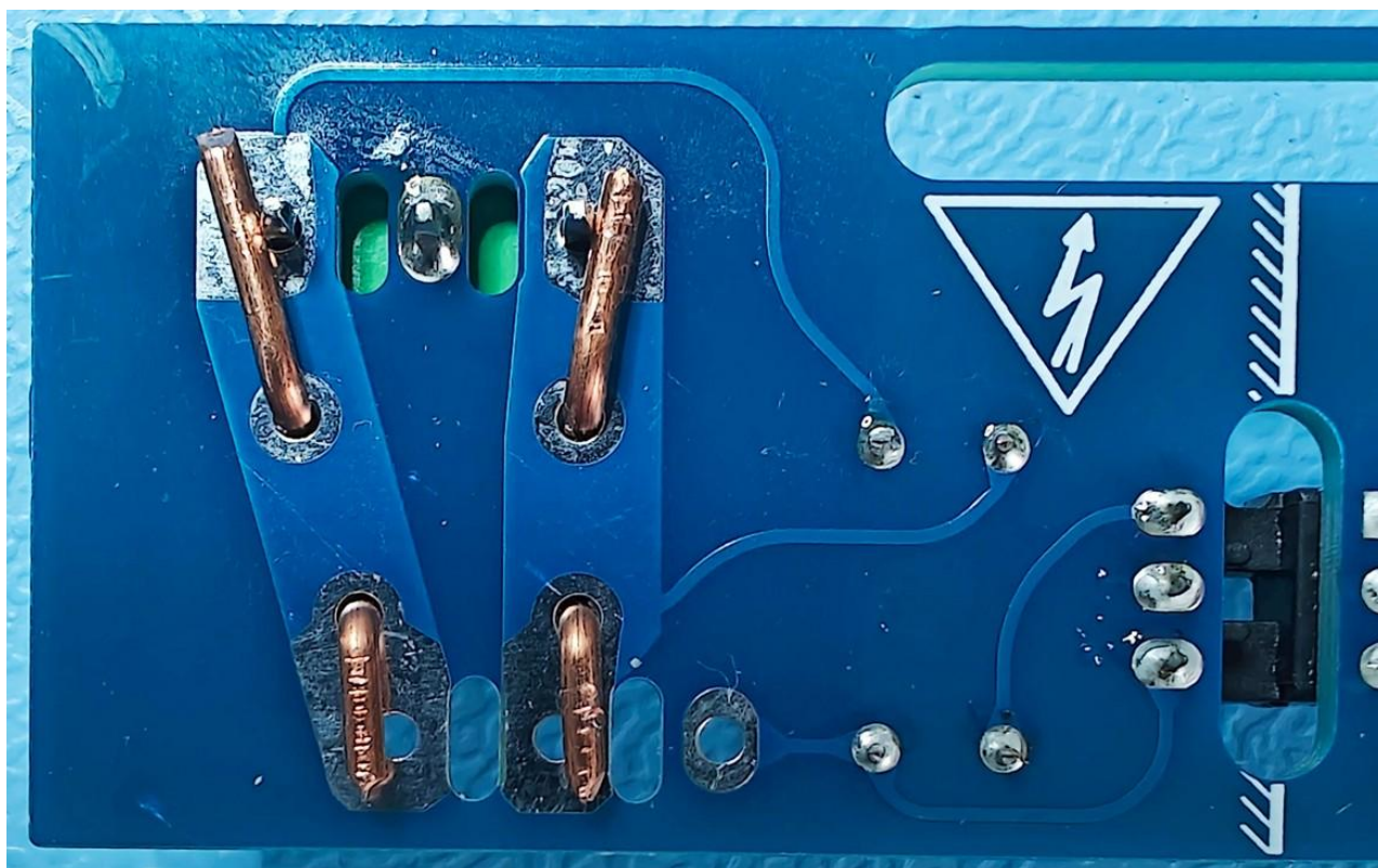
Connecteur de puissance, broche centrale soudée
