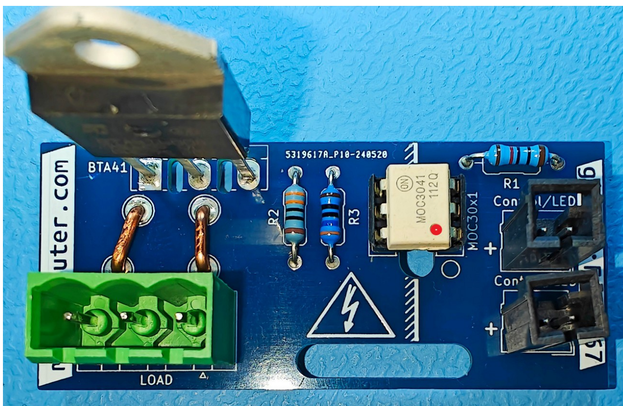
Carte assemblée
