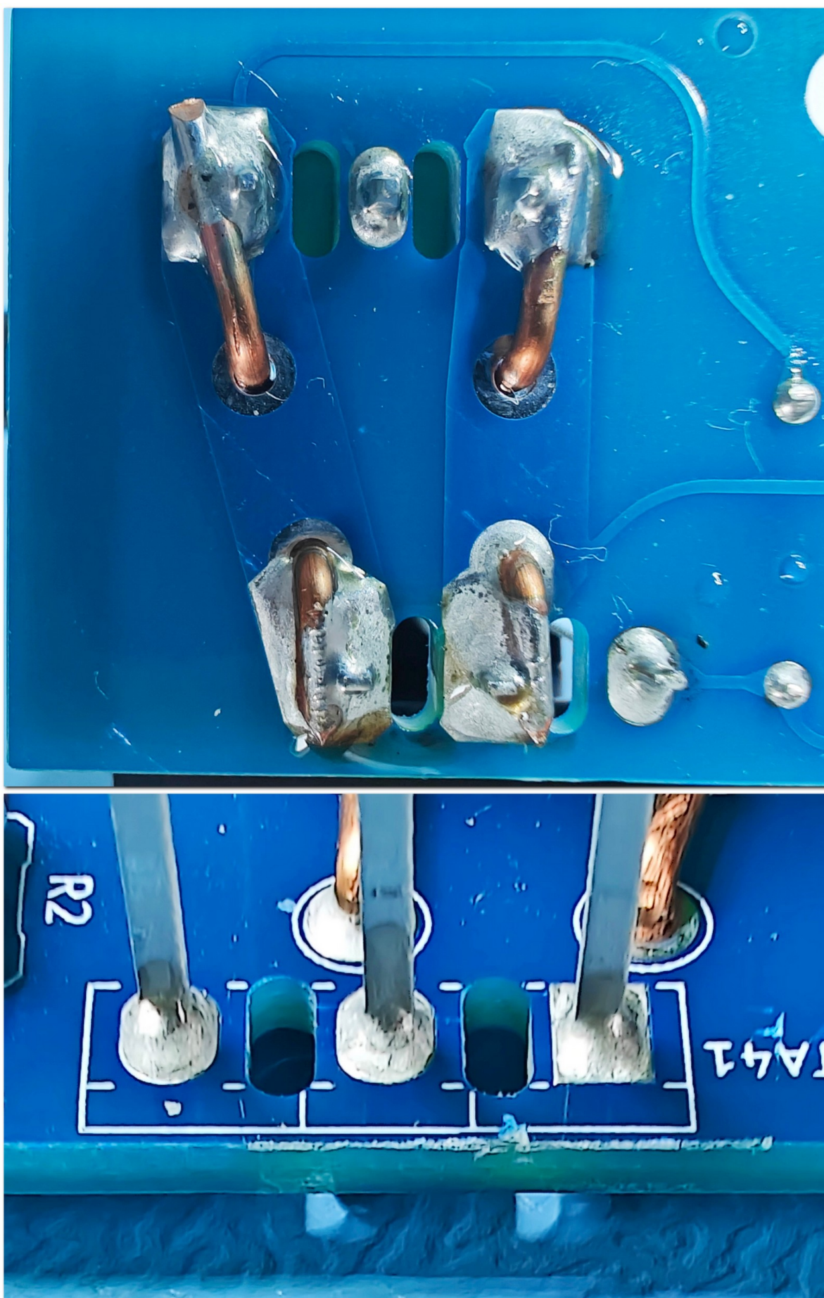
Triac et connecteur soudés
