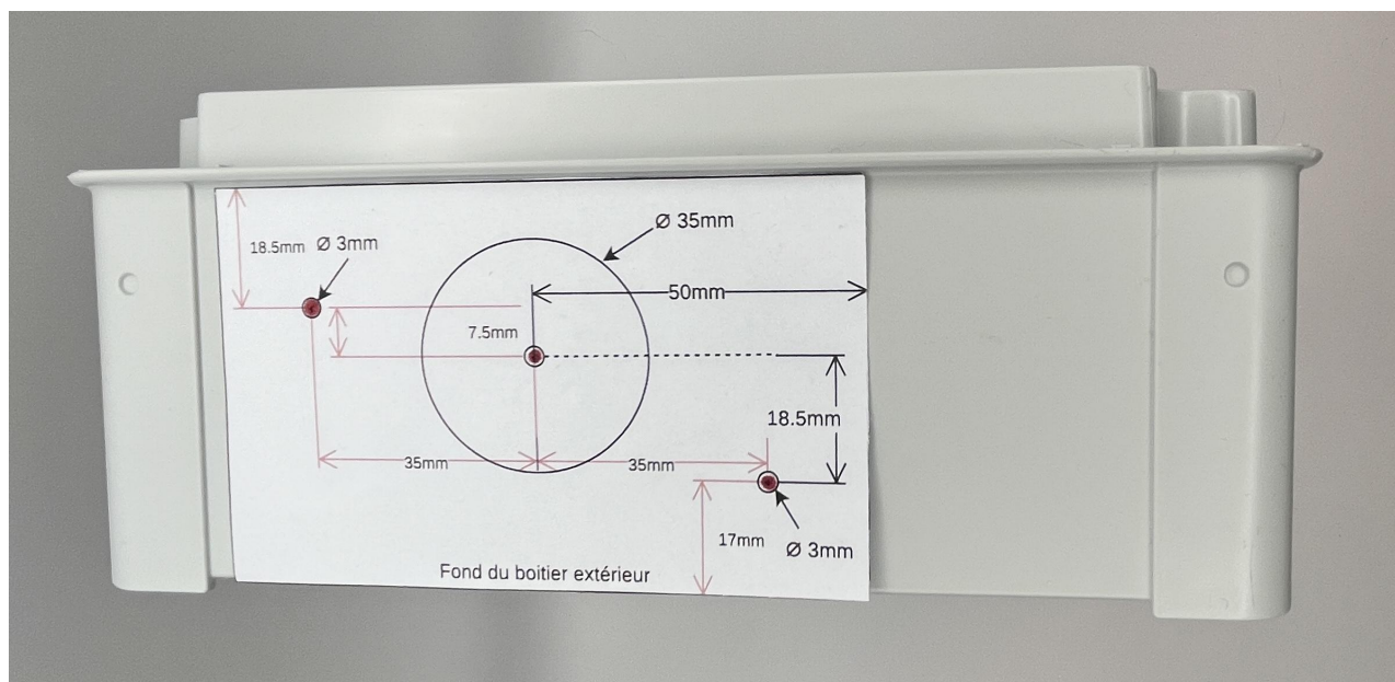
Positionnement du gabarit sur le boîtier
