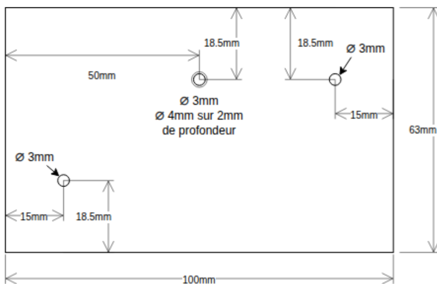
Gabarit de perçage du boîtier
