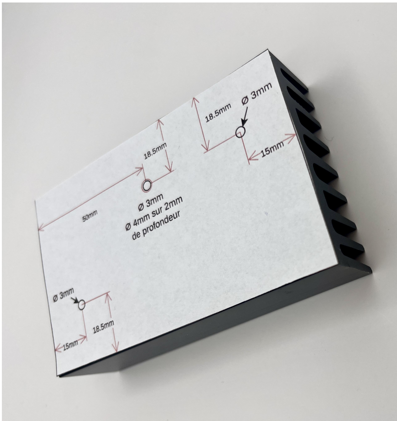
Positionnement du gabarit sur le dissipateur
