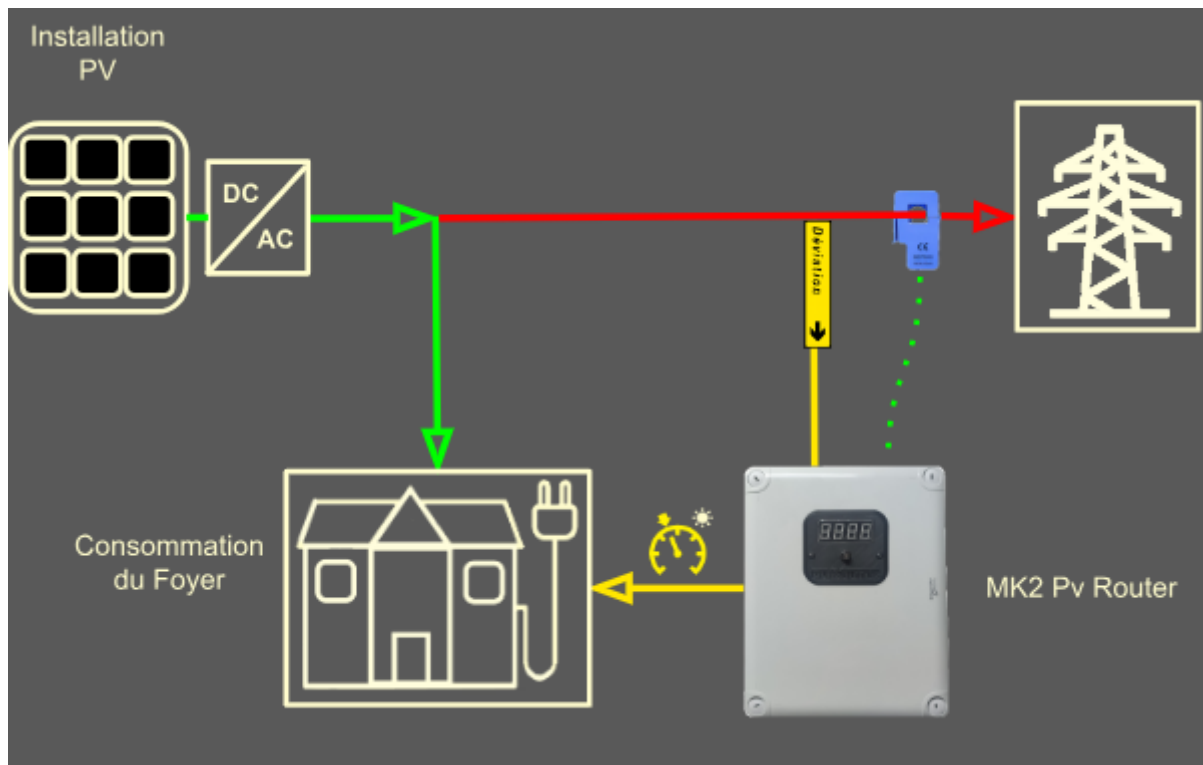
Schéma montrant l'implantation typique du Mk2PVRouter dans une installation domestique.
