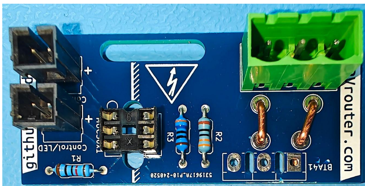
Connecteurs type Molex soudés
