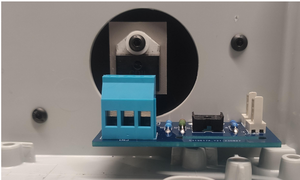
Fixation dissipateur / étage de sortie
