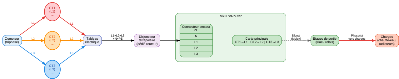
Emplacement des CT — Installation triphasée
