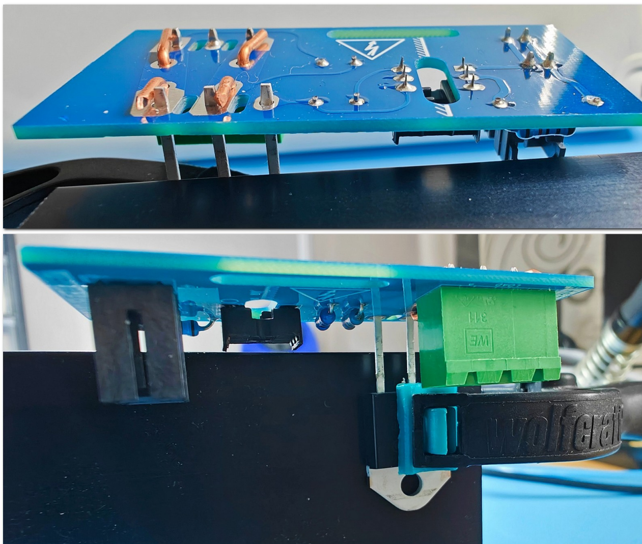
Positionnement du triac
