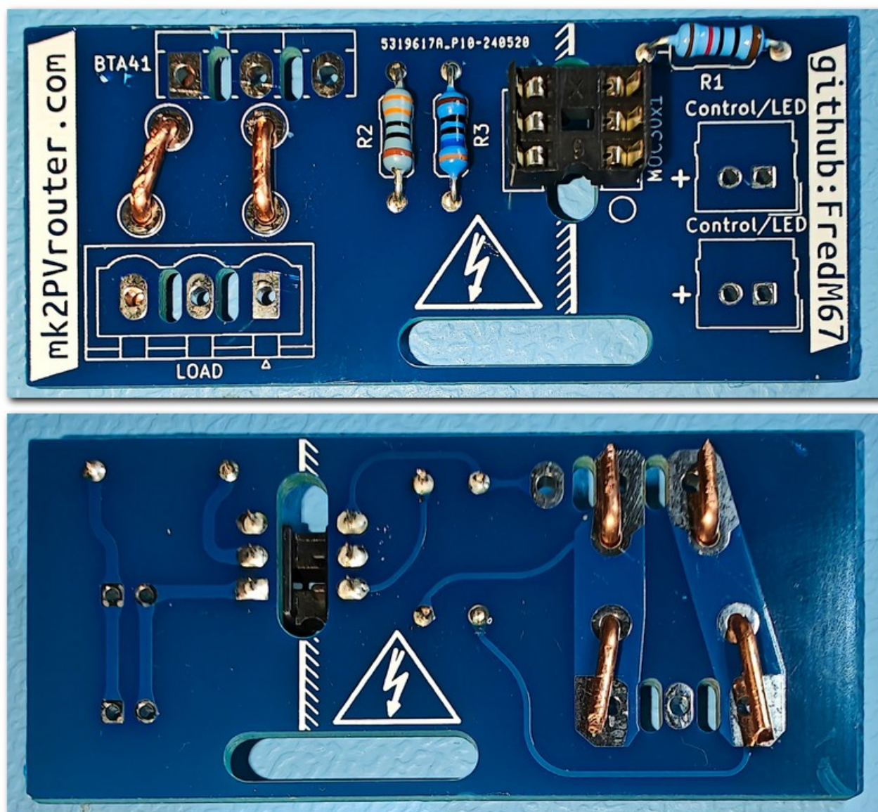
Vue dessus/dessous, résistances et support DIL soudés
