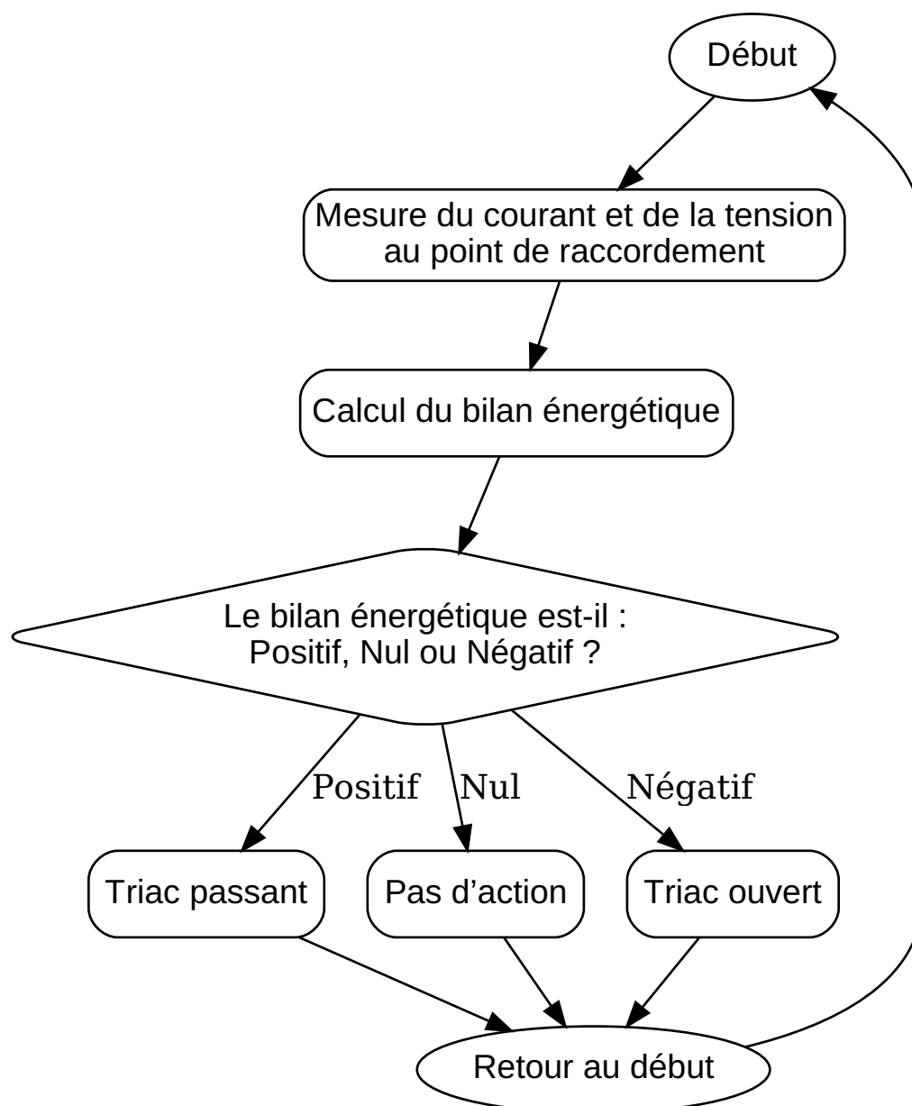
Schéma illustrant le fonctionnement du Mk2PVRouter.
